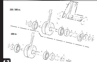
Cigüeñal / Crankshaft GASGAS EC 2004
