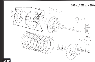
Embrague / Clutch GASGAS EC 2004
