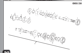
Engranajes cambio / Gear set GASGAS MC 2004
