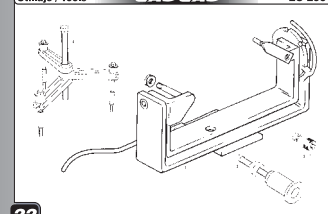
Utilaje / Tools GASGAS EC 2004
