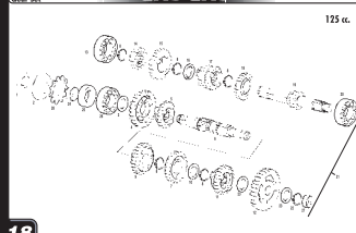
Engranajes cambio / Gear set GASGAS EC 2004
