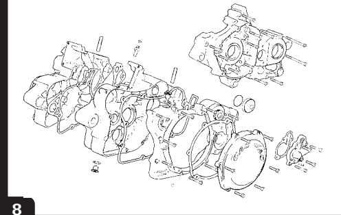
Cárter / Crankcase GAS GAS EC/MC/SM 2006
