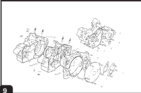
Cárter / Crankcase GAS GAS EC/MC/SM 2006
