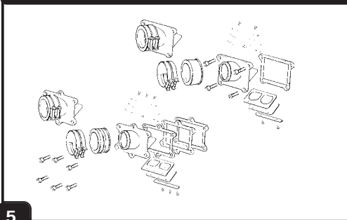
Gaja láminas / Reed valve GAS GAS EC/MC/SM 2006
