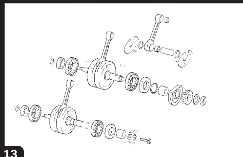
Cigüeñal / Crankshaft GAS GAS EC/MC/SM 2006
