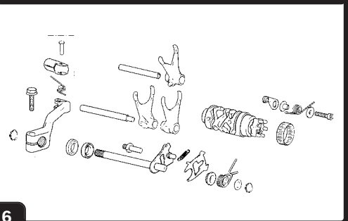
Selector cambio / Shift cam GAS GAS EC/MC/SM 2006
