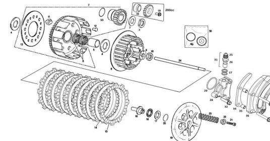
EMBRAGUE CLUTCH
