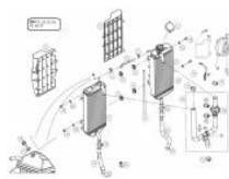
Radiador
