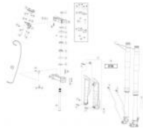
Horquilla
