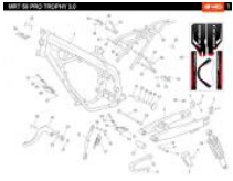
CHASIS
