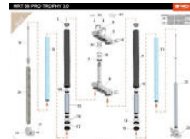
SUSPENSIÓN
