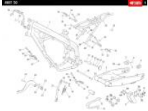
CHASIS
