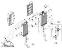
RADIADOR
