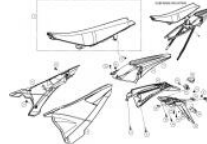
CARENADO TRASERO
