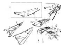
CARENADO TRASERO
