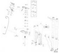
Horquilla
