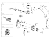
Freno Delantero
