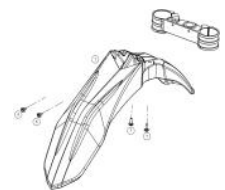
Guardabarros delantero
